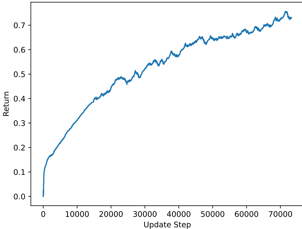
PPO Agent Returns
